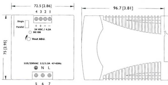
DPP100-24 Dimensions
